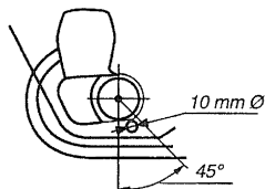
OPEN TRANSMISSION GUARDS GARDE-CHAÎNE OUVERTE
