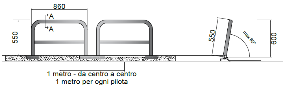
Figura 3.3-1 Cancello di partenza ideale di tipo meccanico (da privilegiare rispetto a quello idraulico)
