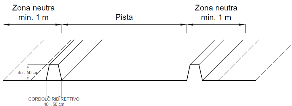
Figura 3.2-1 Sezione pista ideale
